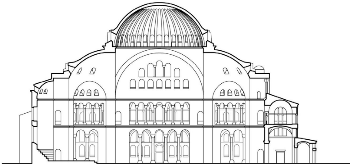
Schnitzzeichnung der Hagia Sophia, Istanbul
