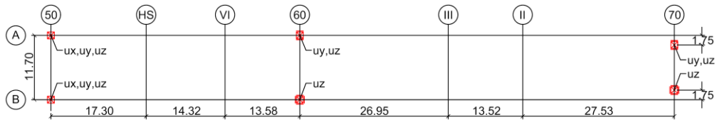
Lagerschema
