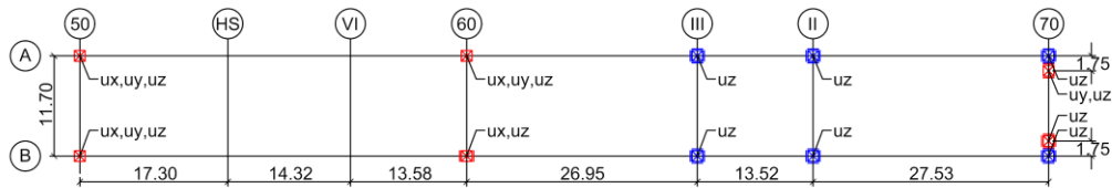
Lagerschema
