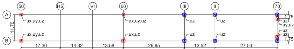
Lagerschema
